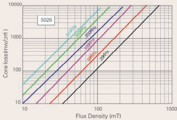
DS铁硅铝系列磁粉心典型磁损耗特性
